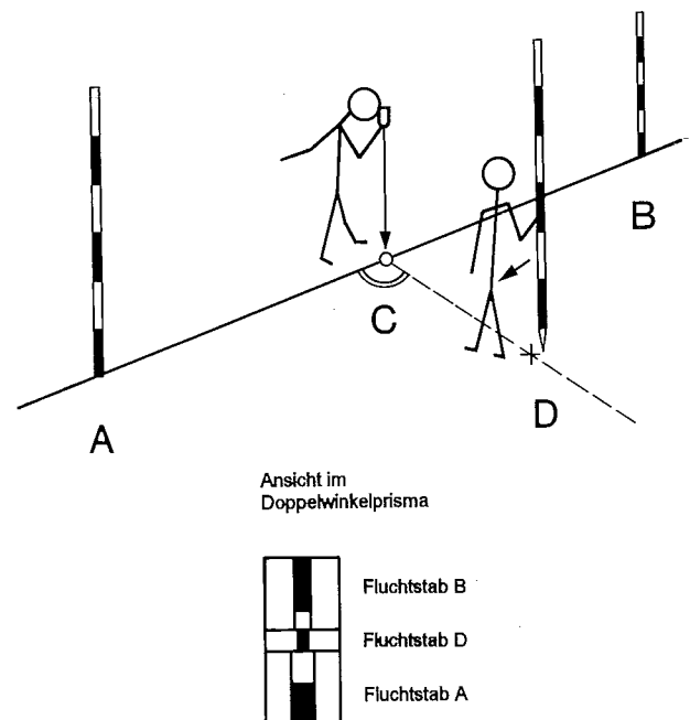
5 Abstecken eines rechten Winkels mit dem Doppelwinkelprisma.
